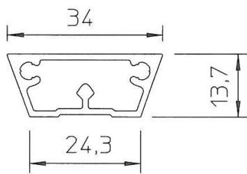
Utanpåliggande spröjs KT991, 995, FD953
